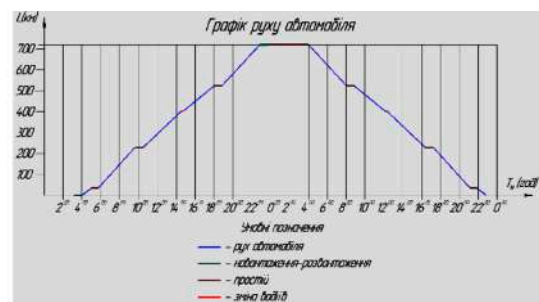
д) графік руху транспортного засобу
